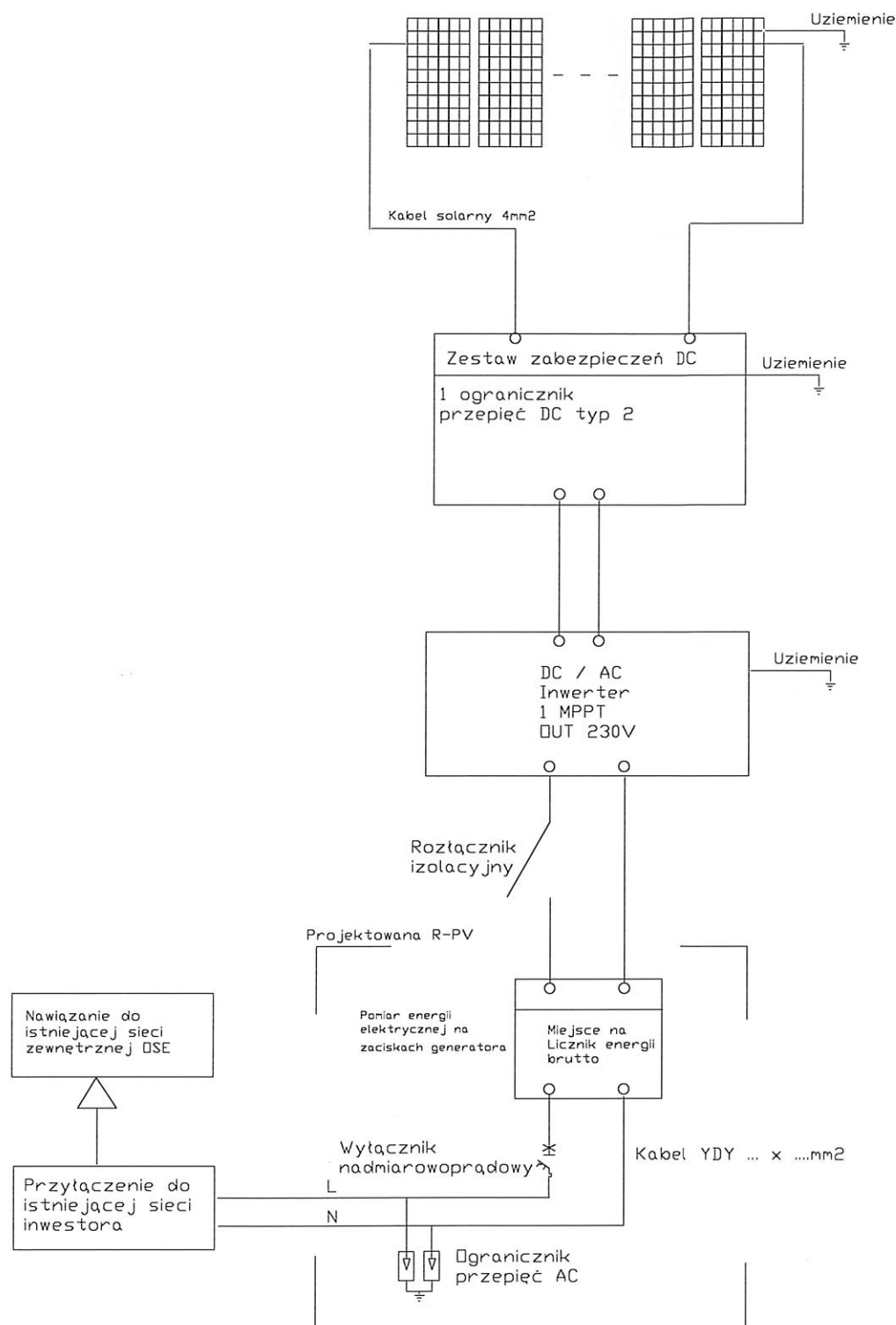
Schemat poglądowy modułów fotowoltaicznych – 2 sekcje
