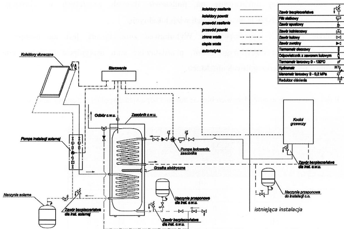
Schemat poglądowy instalacji solarnej dla bud. mieszkalnych
